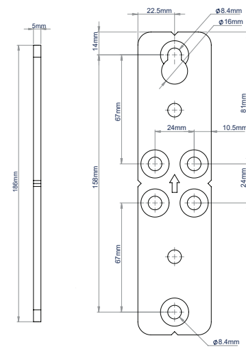
SEITEN-ANSICHT
