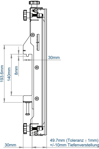
SEITENANSICHT
